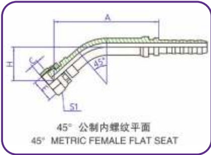
扣压式软管接头 (连接螺母尺寸按BJ1891-77标准)
